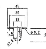
A-A断面図 S=1/2
