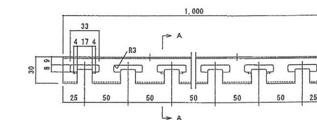
金具図面
