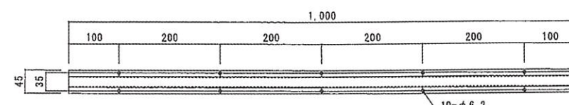
取付穴位置図 S=1/5
